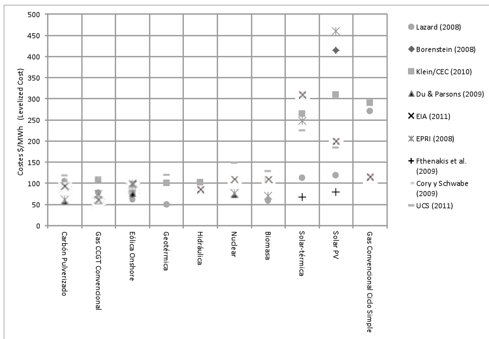
GRÁFICO 6 COSTES ESTIMADOS DE DIVERSAS TECNOLOGÍAS ENERGÉTICAS
